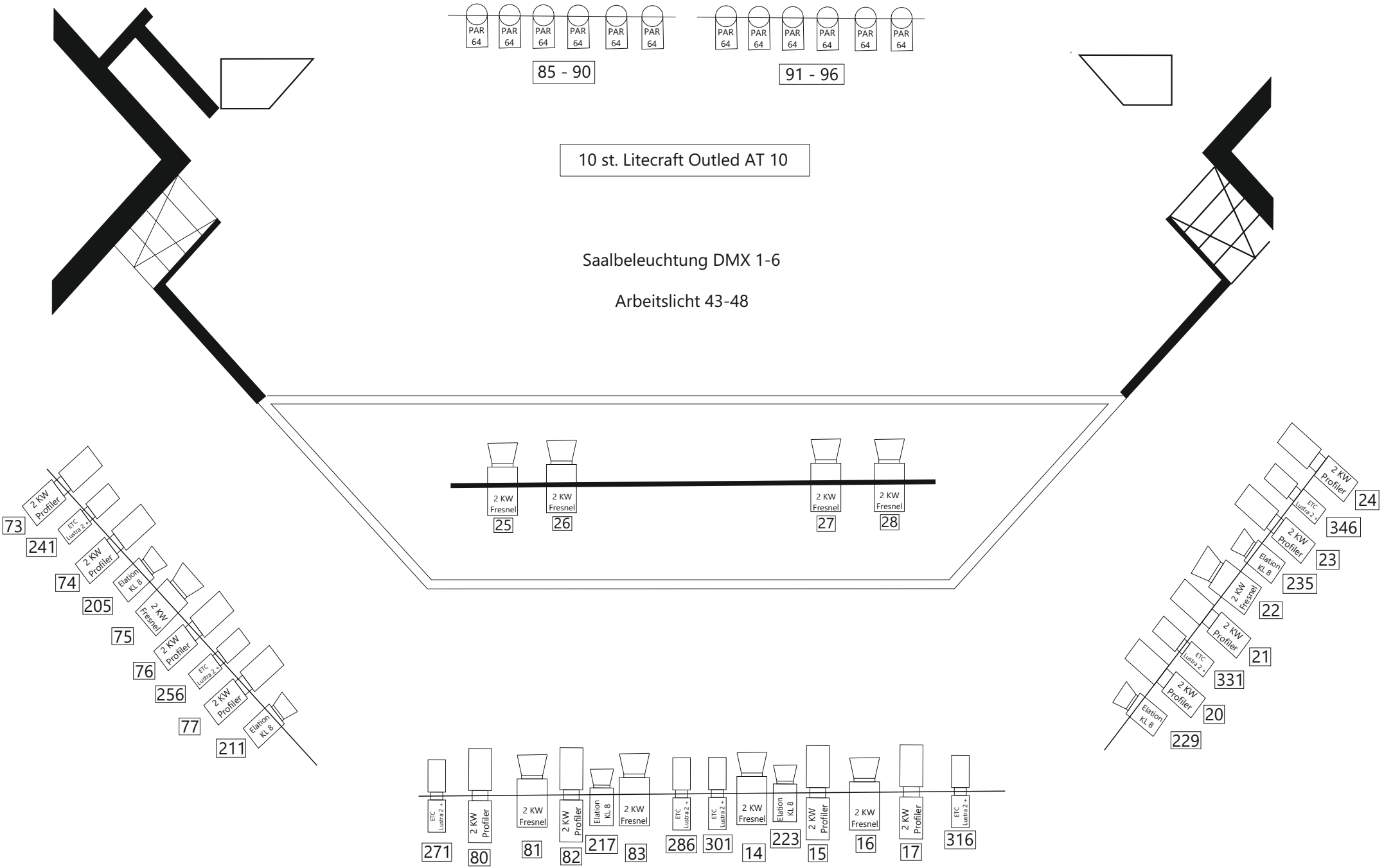
Grundaushang Bürgerhaus Ibbenbüren mit DMX Adressen
